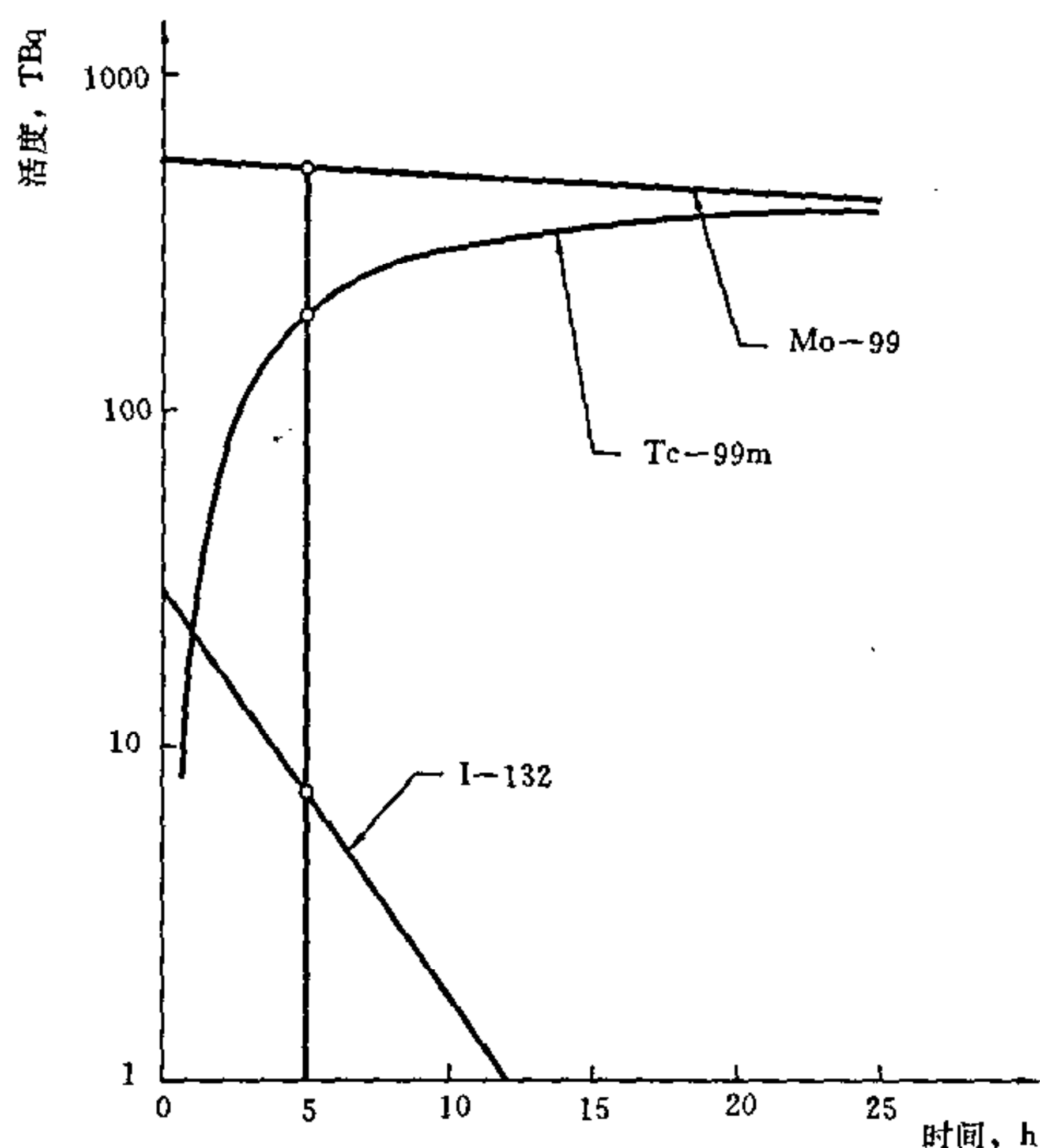
图 C2 ^{99}\text{Mo} 、 ^{99\text{m}}\text{Tc} 、 ^{132}\text{I} 的衰变曲线图
