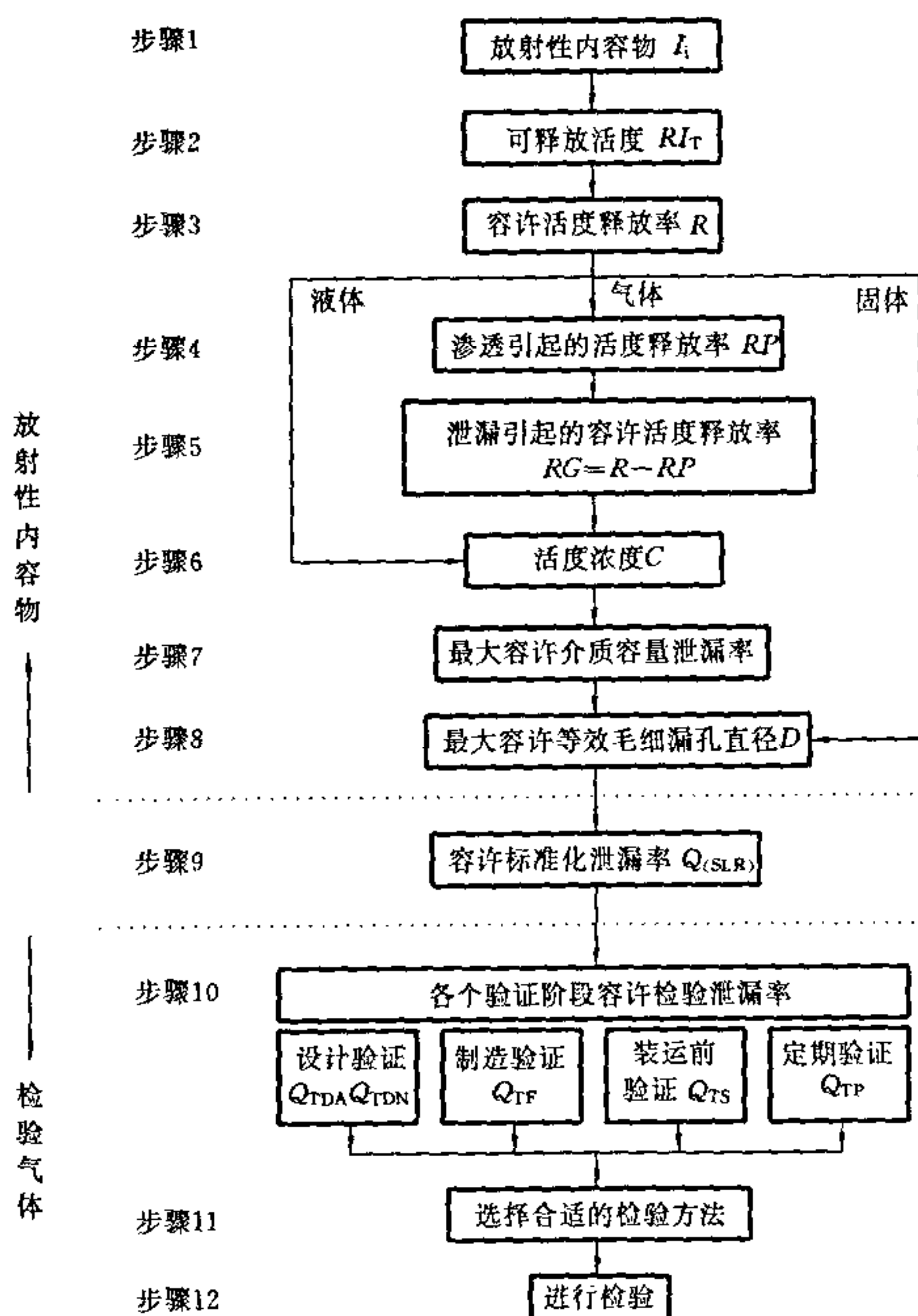
图 1 气体泄漏检验法流程图
